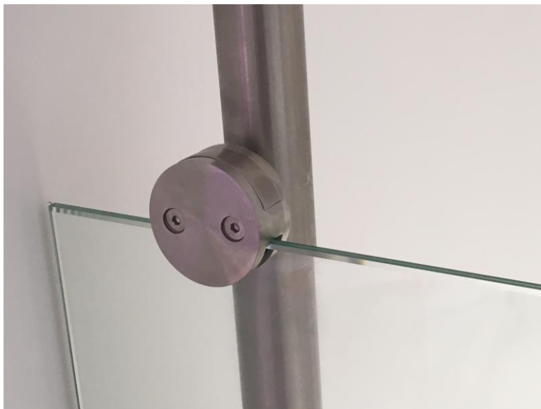
Palier modèle LVB (Lisses plus verre bas)
